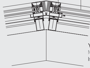
Yatay taşıyıcı profil Profil portant horizontale Profile horizontal bearing
