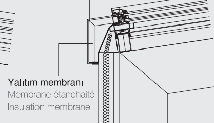
İşıklık Camı 6+16+ (5+5) Vitre de verrière 6+16+(5+5) Glass skylight 6+16+(5+5)
